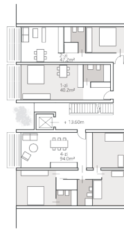
grundriss 4. og 1_200
