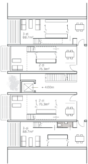
grundriss 1. og 1_200
